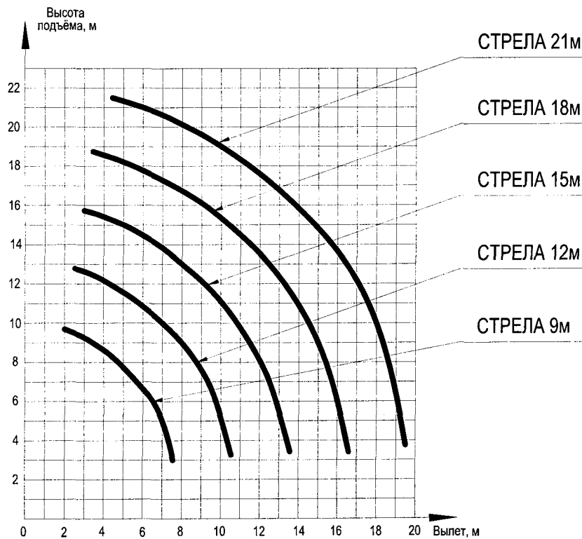
Диаграмма высотных характеристик Рис. 2.5
