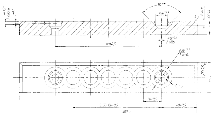
Опора скольжения КС-45724-8.63.102 (Материал БР. АЖ 9-4 ГОСТ 18175-78)
