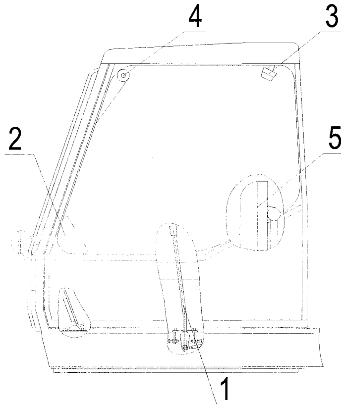
Рис.9.11 Кабина
