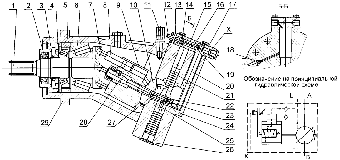
Рис. 9.24 Гидромотор регулируемый
