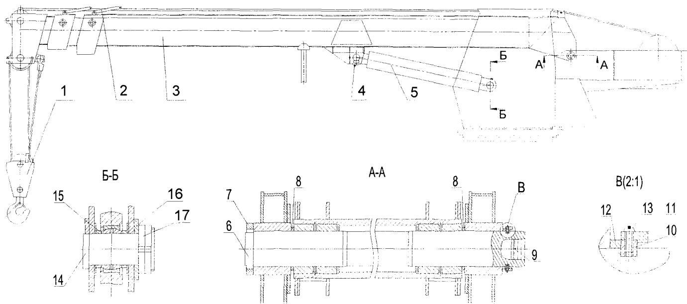
Рис. 9.13 Рабочее оборудование
