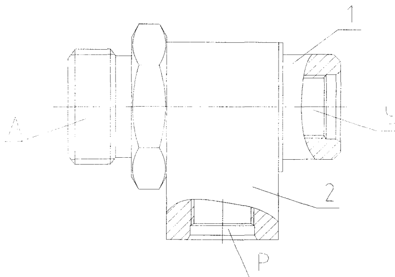
Рис. 9.37 Гидрозамок
