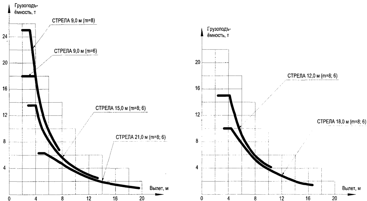
Диаграмма грузových характеристик Рис. 2.1
