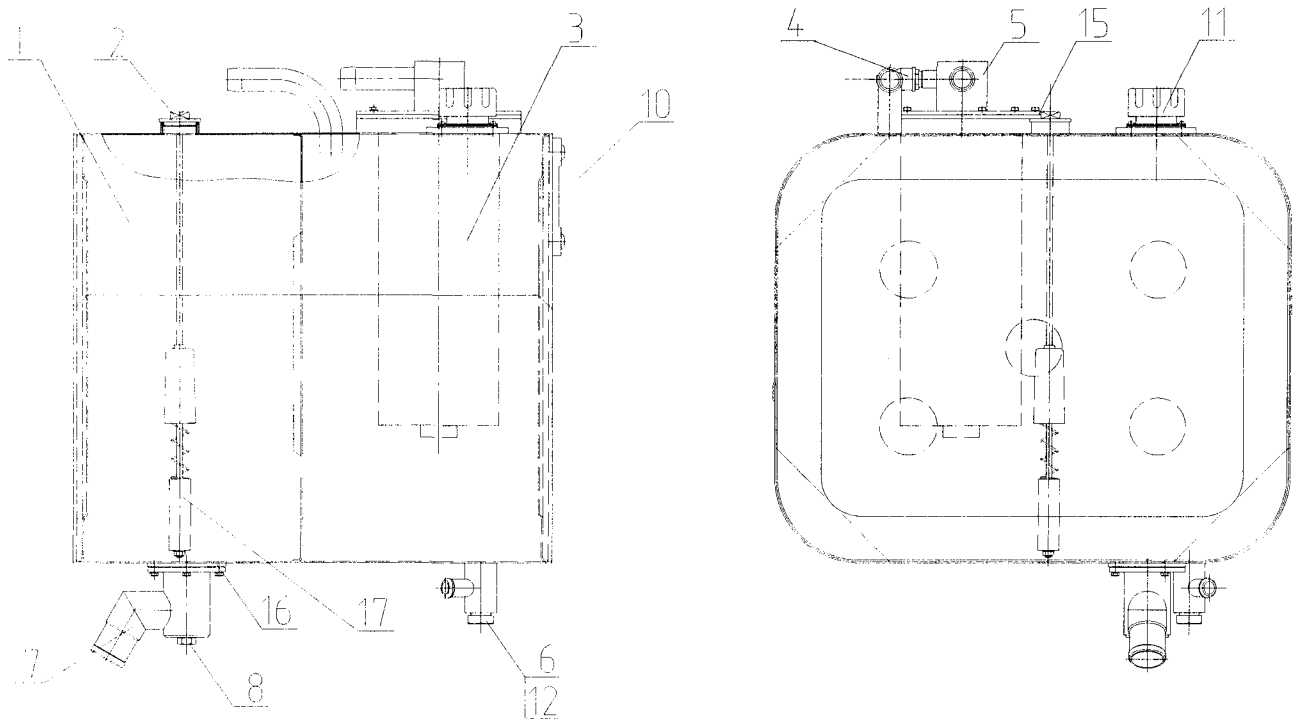
Рис. 9.22 Гидробак
