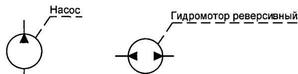
Рис. 9.23 Насос - гидромотор
