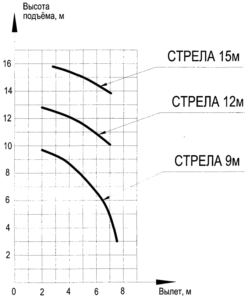
Диаграмма высотных характеристик Рис. 2.7
