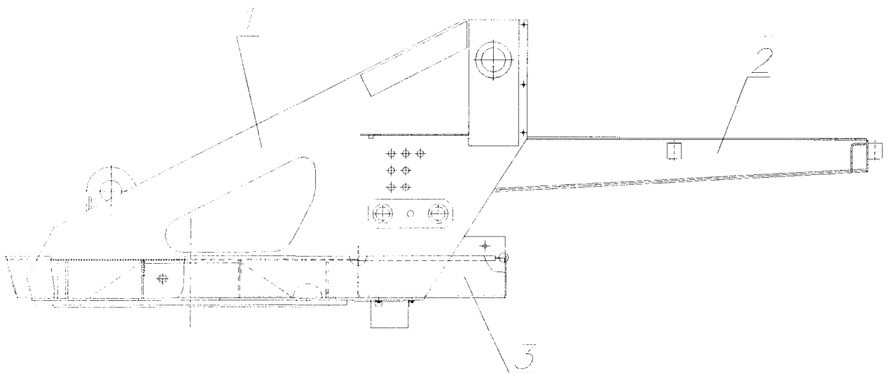
Рис. 9.7 Рама поворотная
