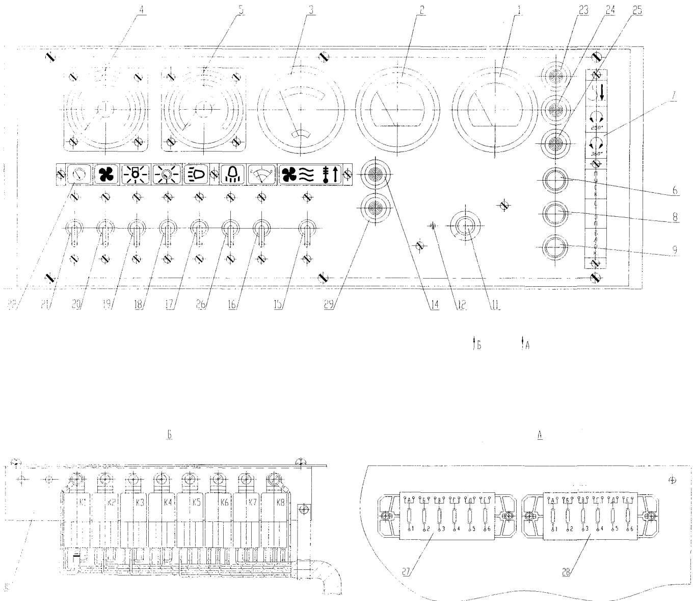
Рис. 9.52 Щиток приборов
