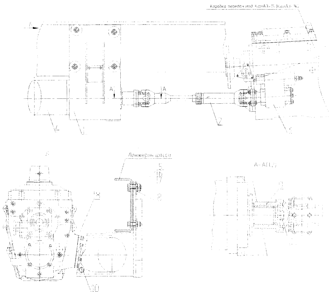
Рис.15.1 привод насоса
