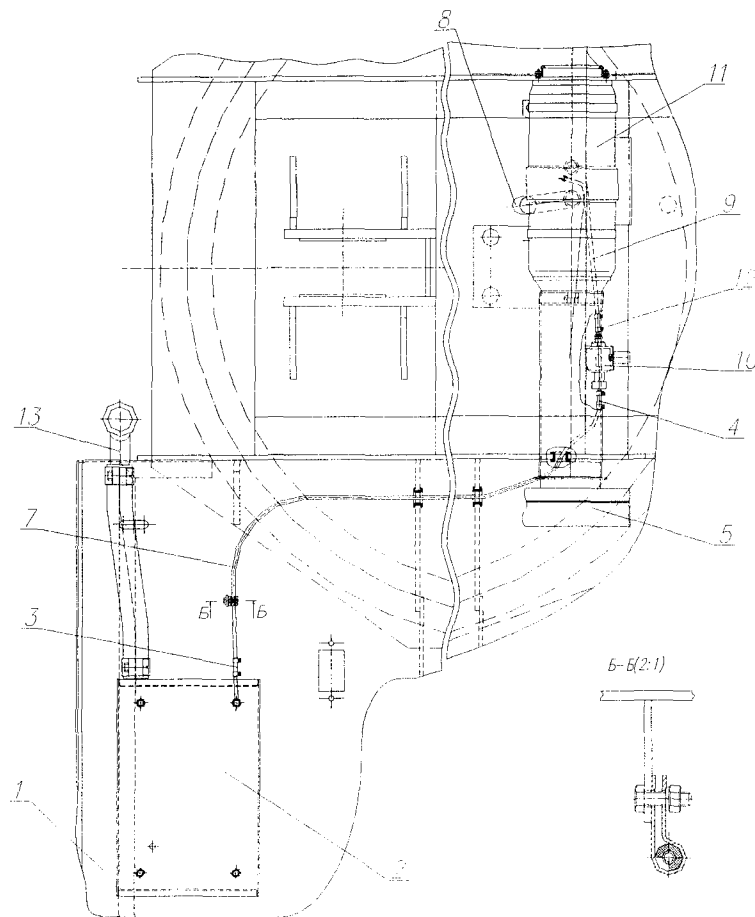
Рис. 9.12 Отопительная установка
