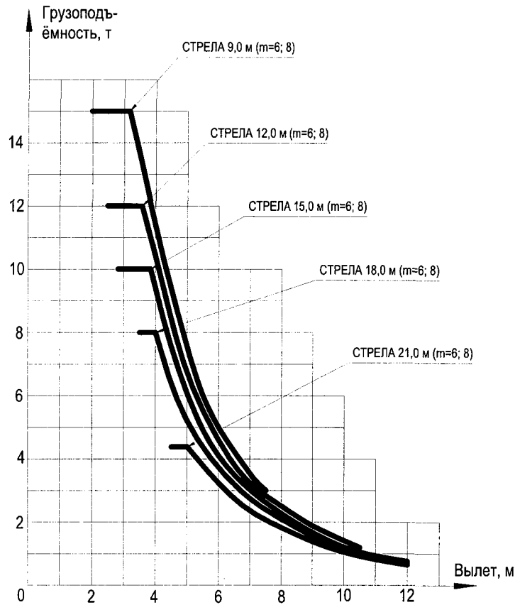
Диаграмма грузовых характеристик Рис. 2.2
