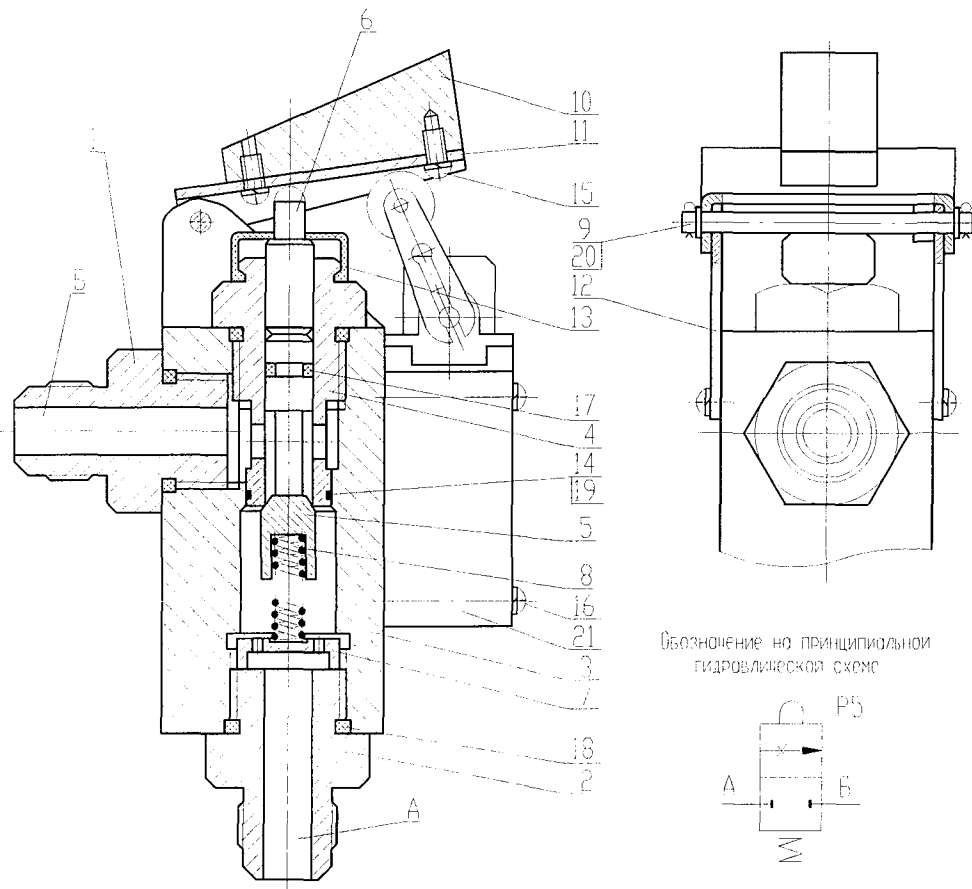
Рис. 9.31 Кран затяжки крюка
