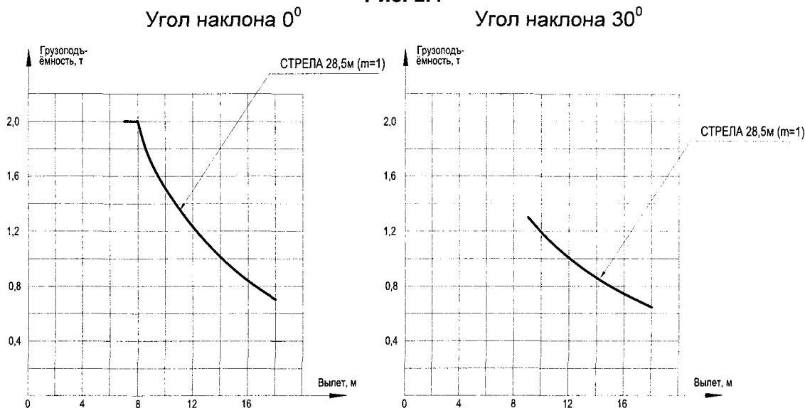
Диаграмма грузовых характеристик Рис. 2.4
