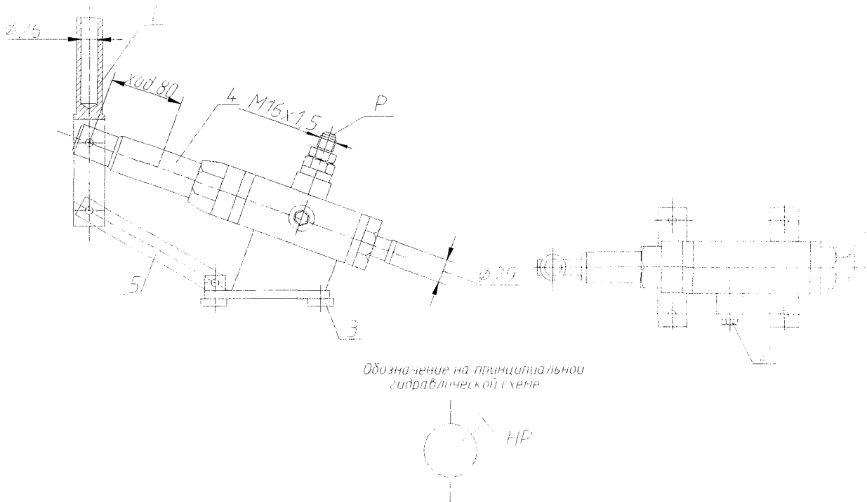
Рис. 9.25 Ручной насос
