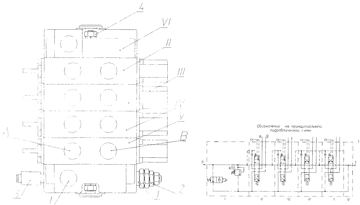
Рис. 9.33 Гидрораспределитель поворотной части
