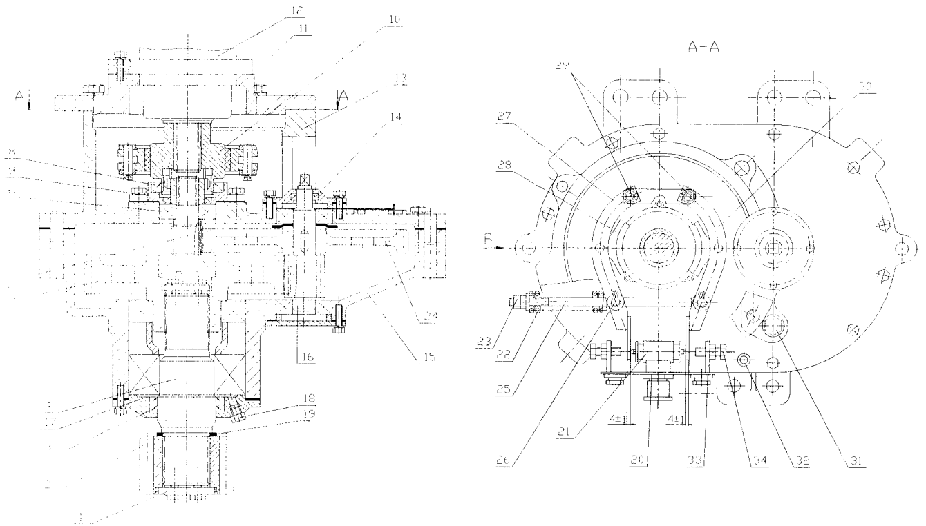
Рис. 9.10 Механизм поворота
