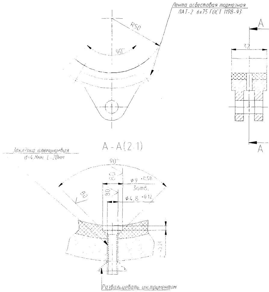
КС-2574.28.130 Колодка
