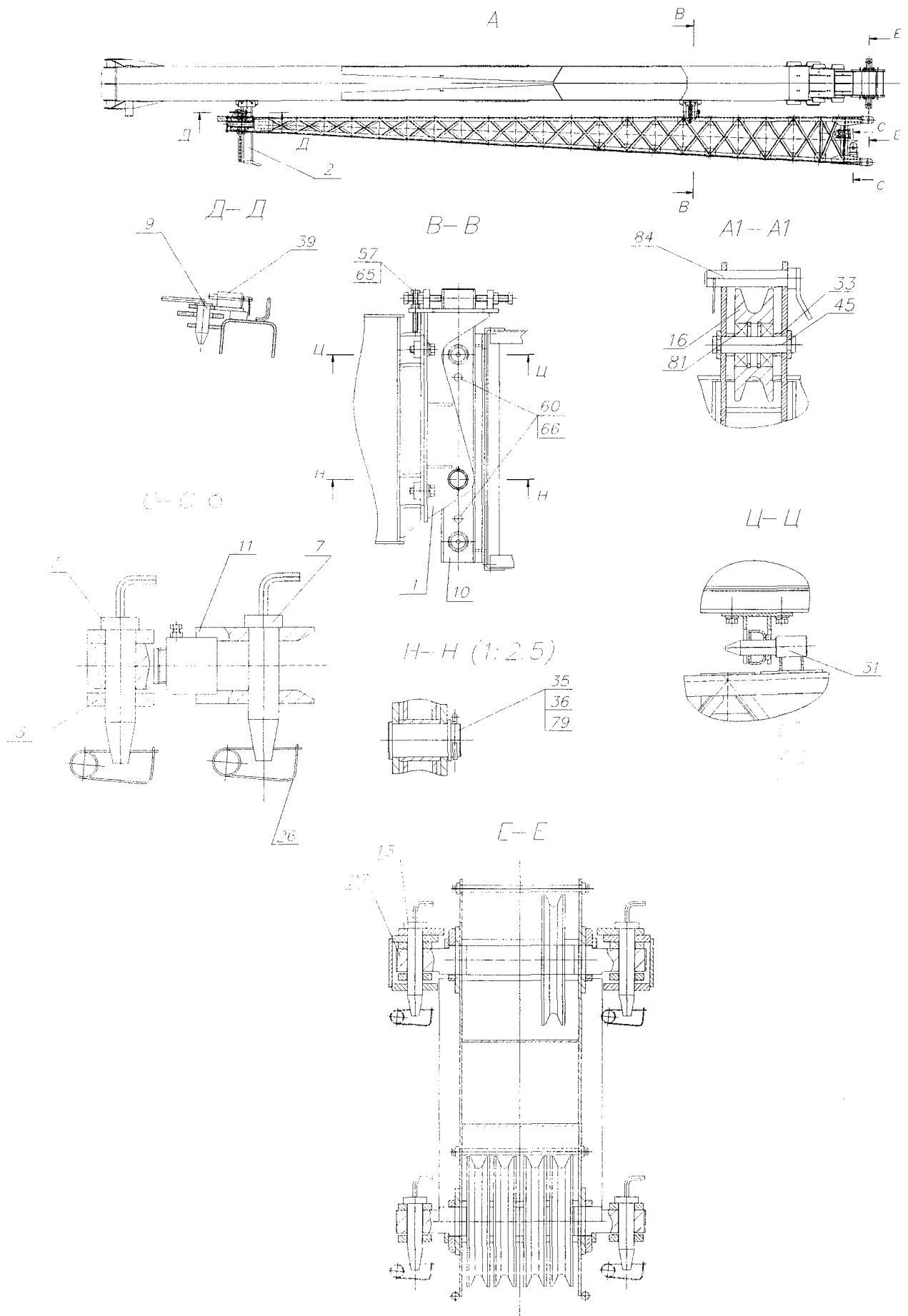
Рис. 9.16. лист 2 Гусёк
