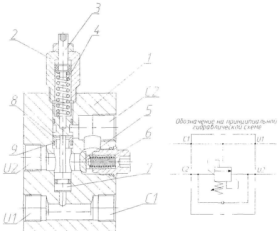
Рис. 9.35 Тормозной клапан грузовой лебёдки
