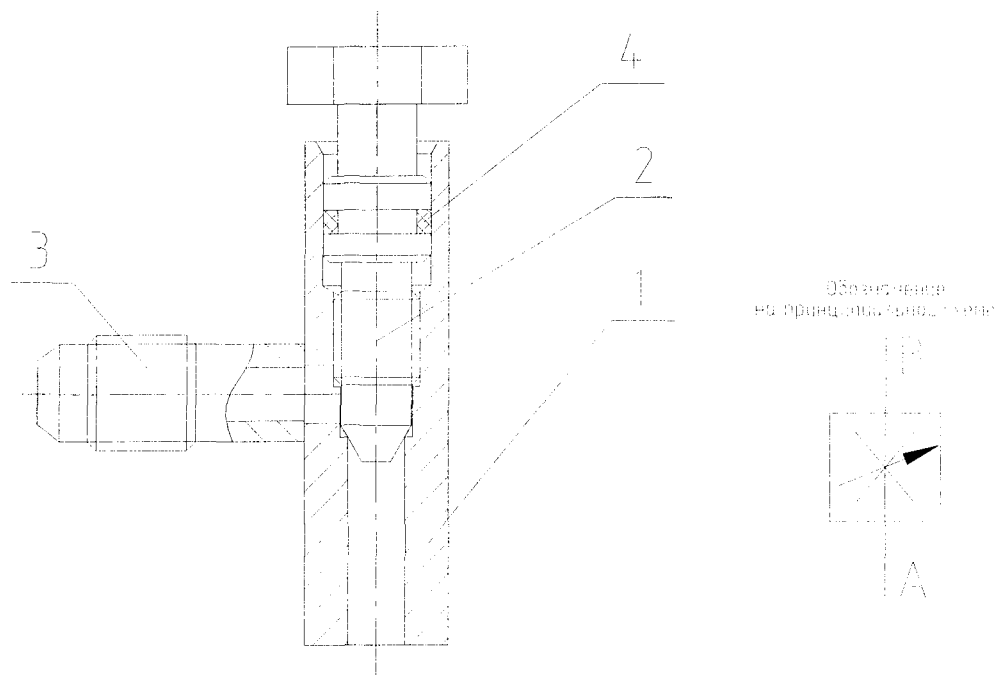
Рис. 9.39 Вентиль-дрессель (разогревочный)
