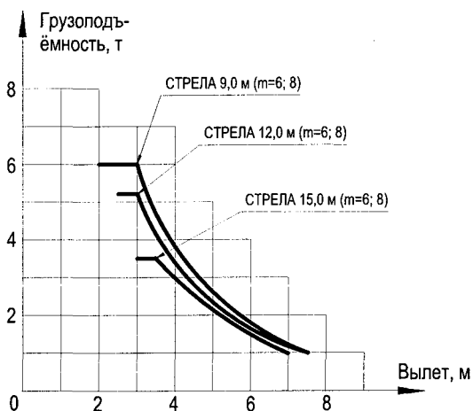
Диаграмма грузовых характеристик Рис. 2.3
