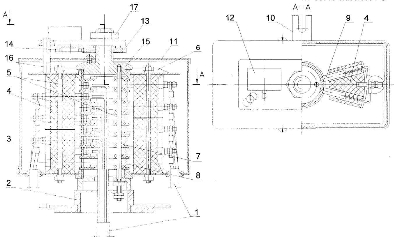
Рис. 9.48 Токосъёмник
