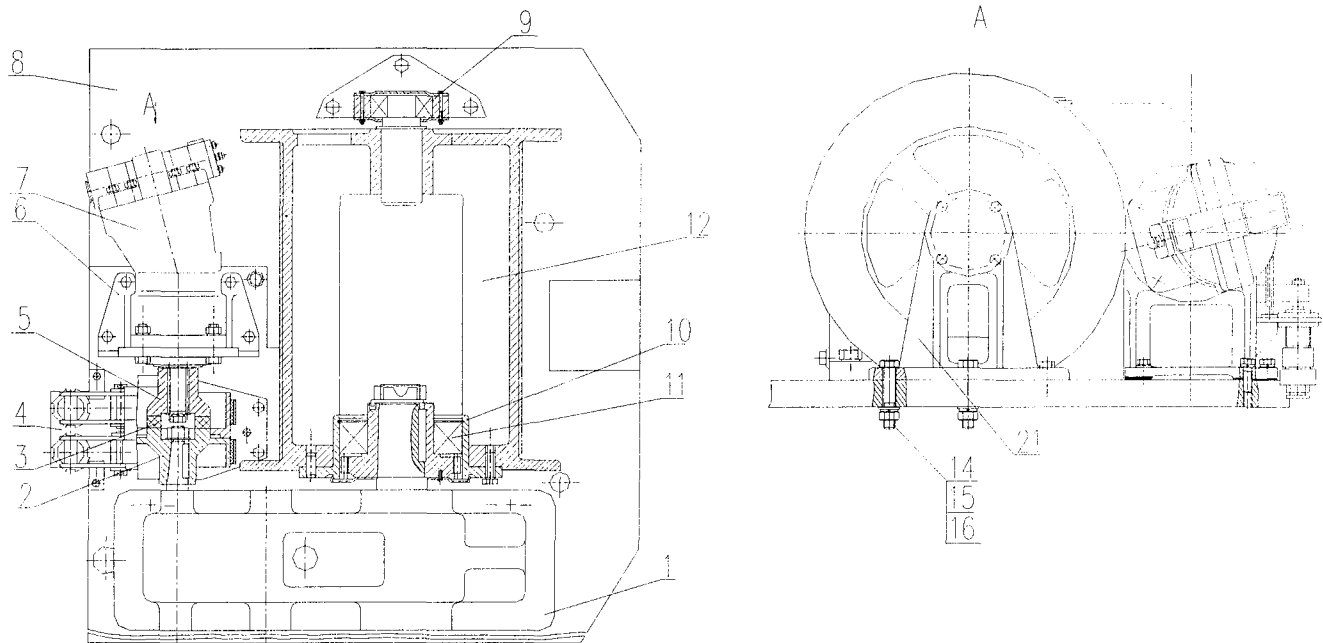
Рис. 9.8 Грузовая лебёдка
