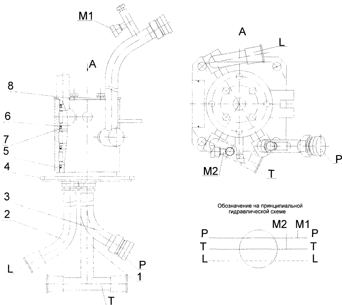
Рис. 9.42 Вращающееся соединение
