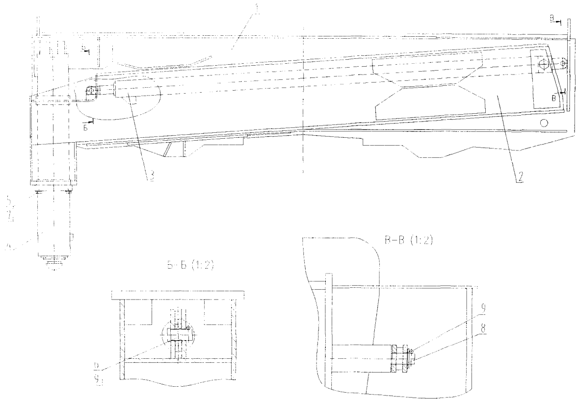
Рис. 9.3 Опора выдвижная
