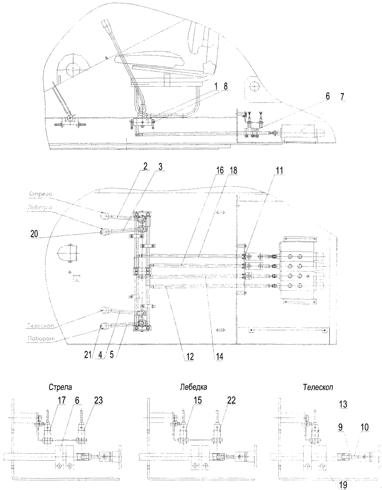
Рис. 9.20 Привод управления крановыми операциями
