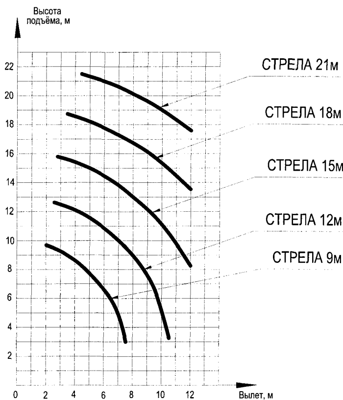
Диаграмма высотных характеристик Рис. 2.6
