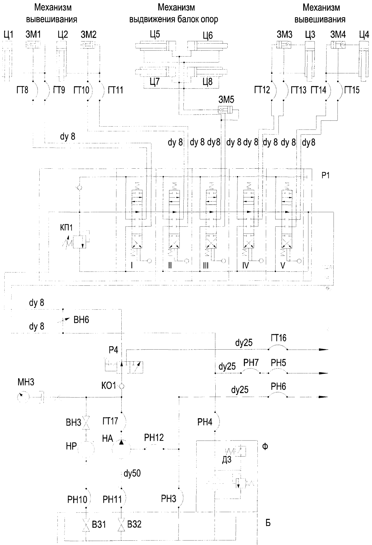
Рис. 9.21 лист 1 Схема гидравлическая принципиальная неповоротной части
