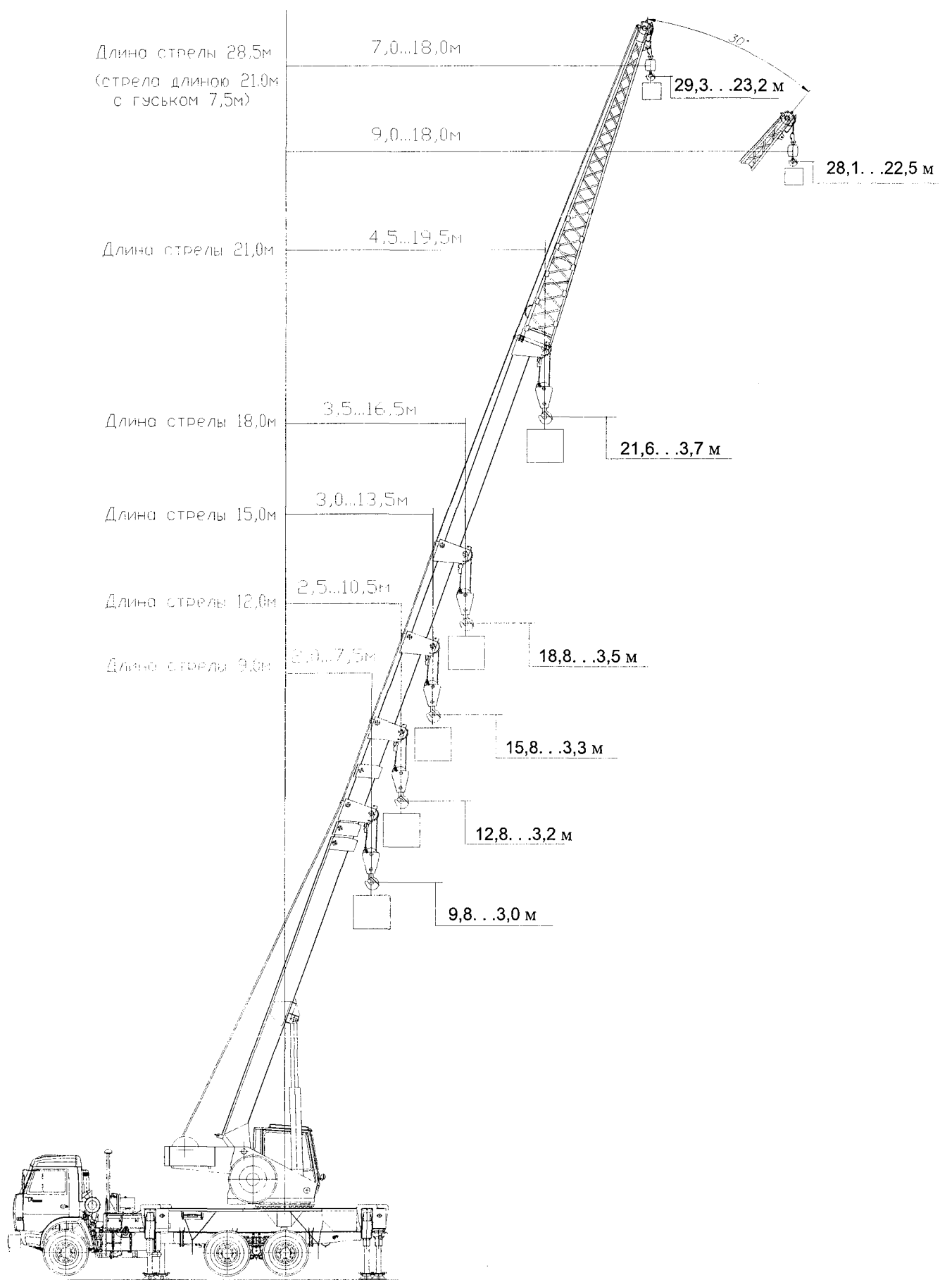
Рис. 1.1 Общий вид крана в рабочем положении с грузом
