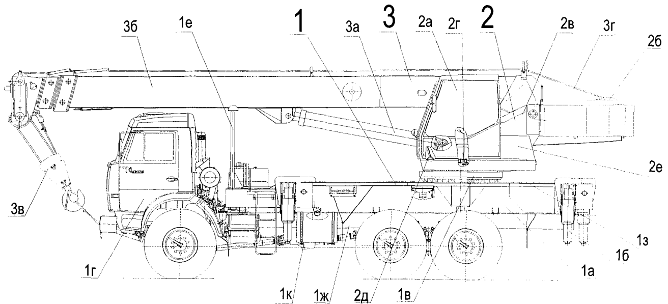
Рис. 9.1. Кран стреловой автомобильный
