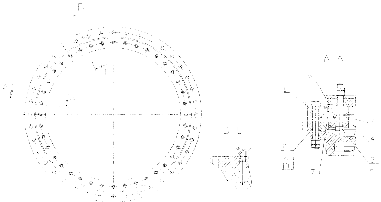
Рис. 9.4 Опора поворотная
